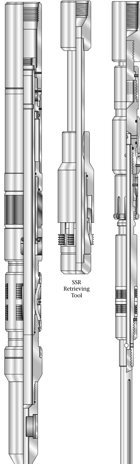
SSR-WS Packer
